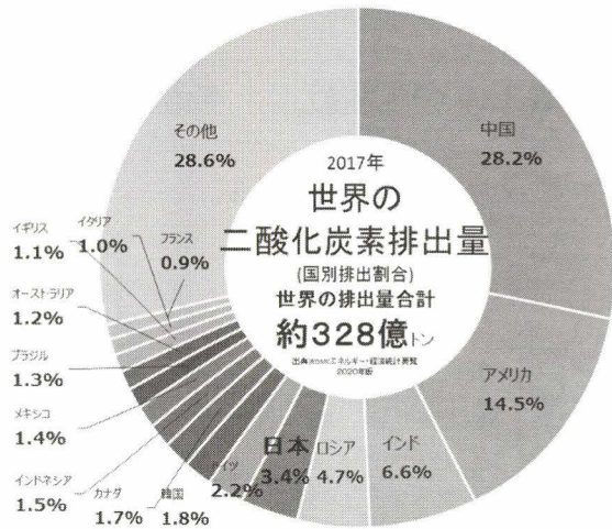
図表 8 世界のエネルギー起源 CO 2 排出量（2017 年）
