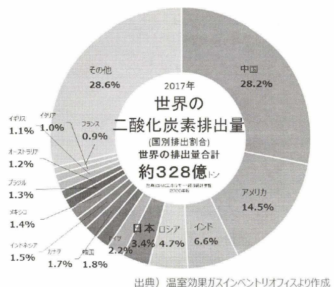
世界のエネルギー起源CO2排出量(※2)
