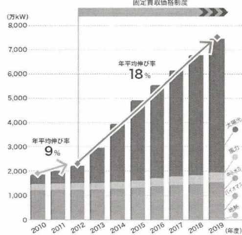
再エネの設備容量の推移(大規模水力は除く)(※1)
