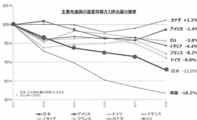
主要先進国の温室効果ガス排出量の推移(※1)
